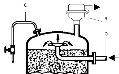
a = Be- und Entlüfter b = Rohwasserleitung c = Entlüftungsleitung
