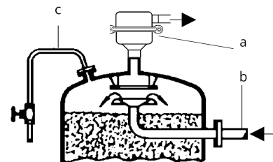
a = Be- und Entlüfter b = Rohwasserleitung c = Entlüftungsleitung
