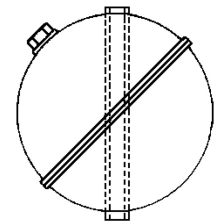
SC 8 mit Innenrohr und Füllschraube, für drucklose Behälter
