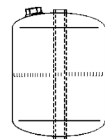
SC 8 mit Innenrohr und Füllschraube, für drucklose Behälter
